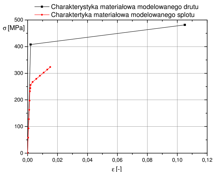
Rys. 4. Charakterystyki materiałowe modeli siatki gabionowej
