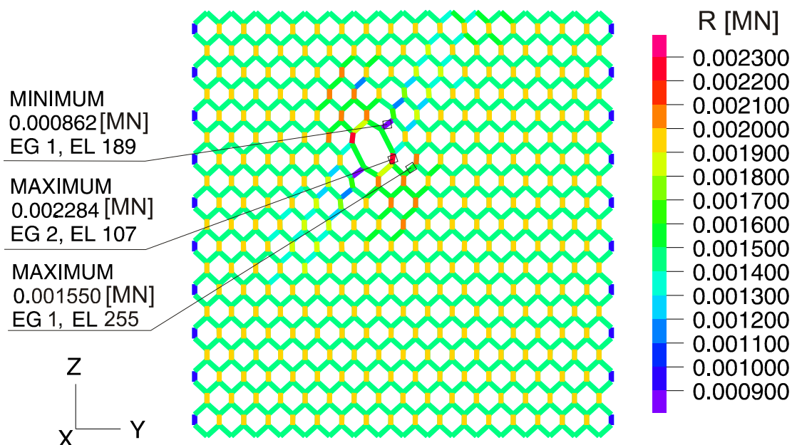
Rys. 7. Warstwicę sił wewnętrznych elementów modelu siatki gabionowej z pojedynczym defektem uzyskane dla maksymalnej dopuszczalnej wartości obciążenia rozciągającego siatkę
