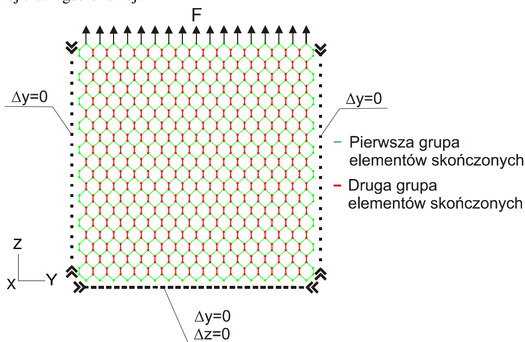
Rys. 5. Siatka MES modelu siatki gabionowej (trzeci etap obliczeń)
